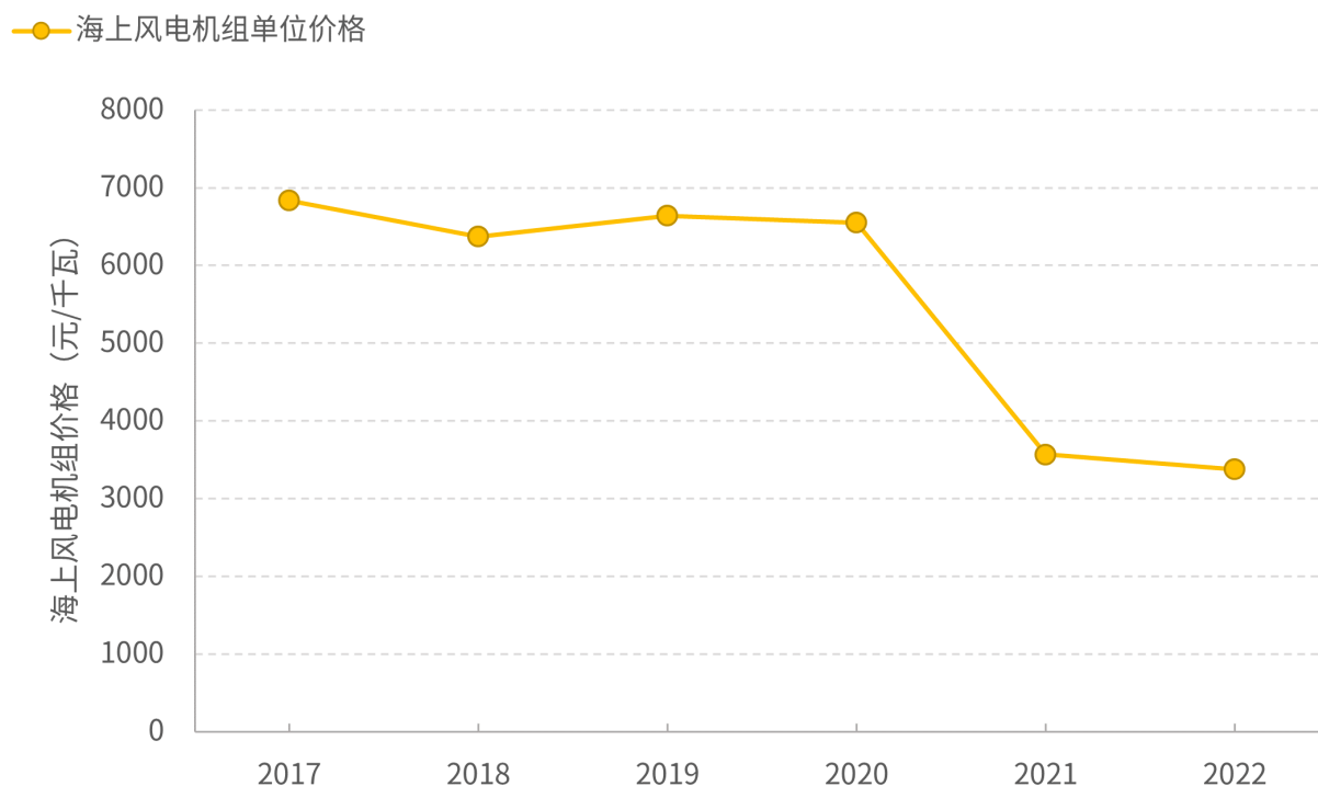
图 2.10 2017-2022 年我国海上风电机组单位千瓦价格（数据来源：CWEA）
