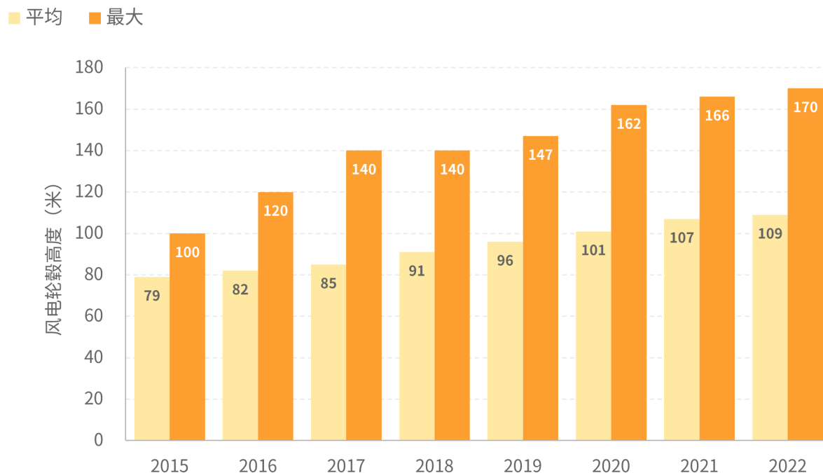
图 2.4 2015-2022 我国新增风电机组平均和最大轮毂高度 (数据来源: CWEA)
