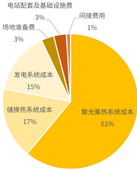
图 4.3 青海中控德令哈 50 兆瓦塔式太阳能热发电站建造成本组成 (国家太阳能光热产业技术创新战略联盟等, 2022)
