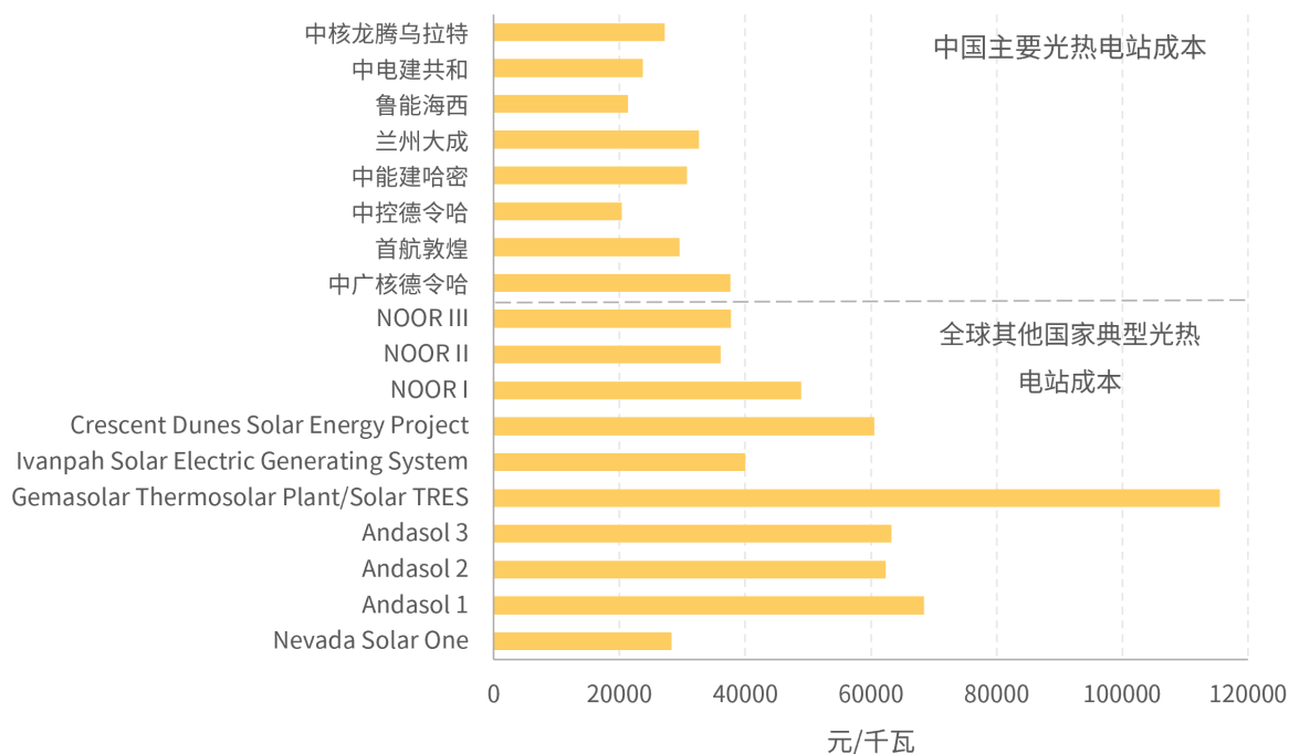
图 4.5 我国与世界典型光热电站成本对比
